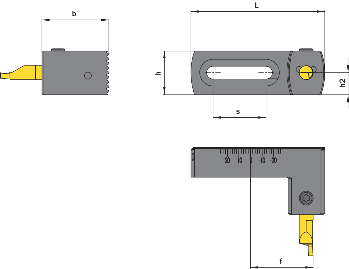
Abbildung zeigt / Drawing shows: MOS.STK.A06.A
