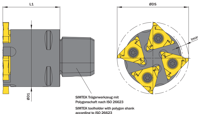
Abbildung zeigt / Drawing shows: M80.C450.40.04
