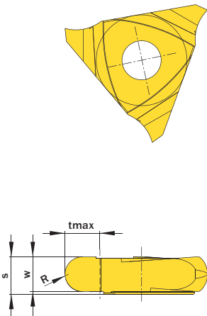
Abbildung zeigt / Drawing shows: M14.0500.250 VR
